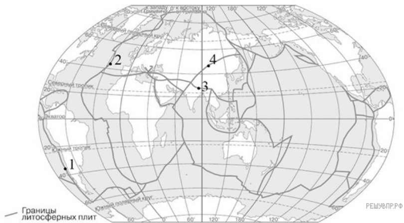
Границы литосферных плит
